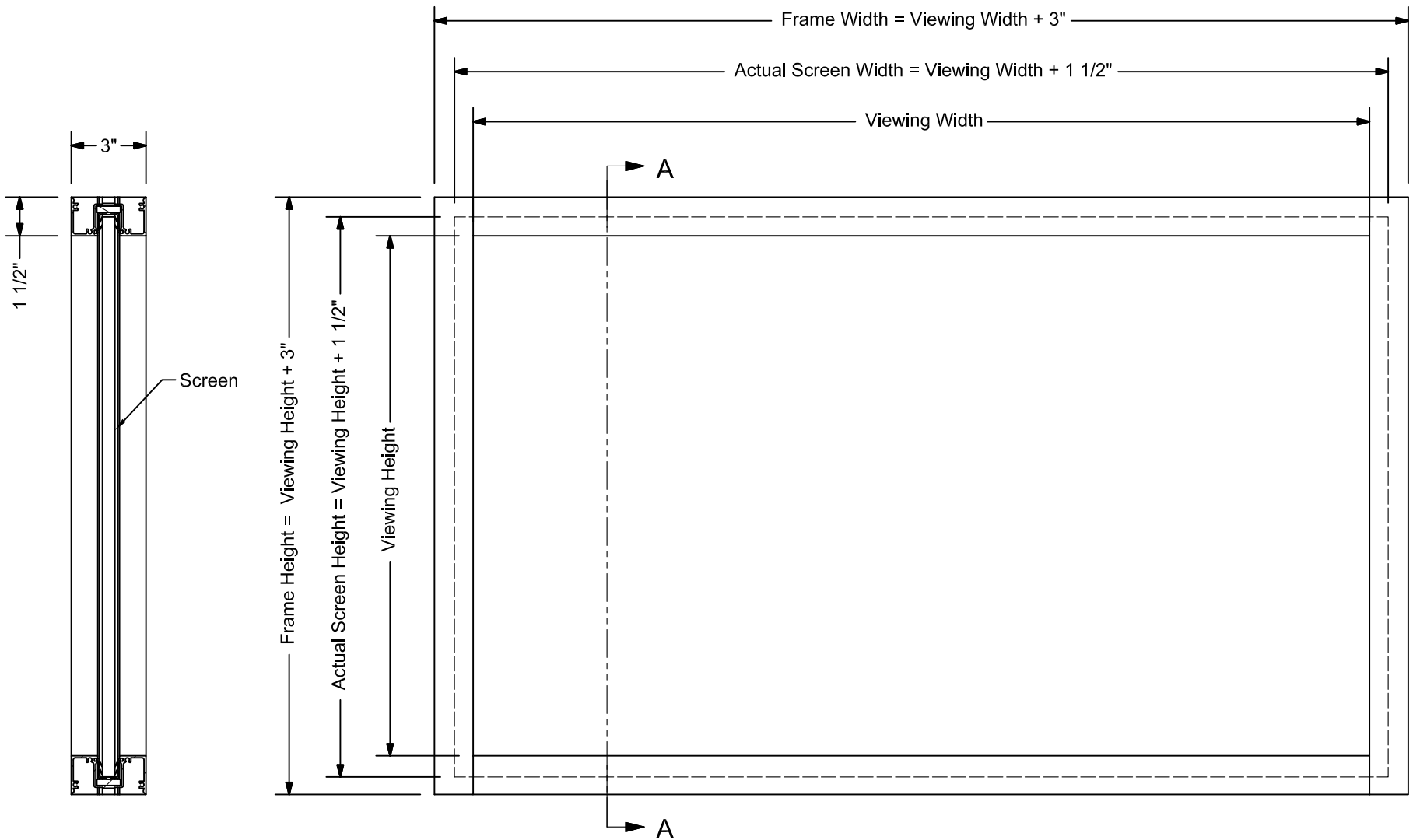
SECTION A-A
